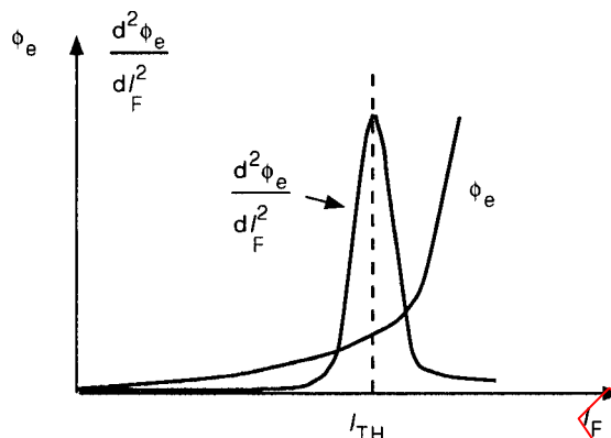
Figure 5 – Courant de seuil d'une diode laser
