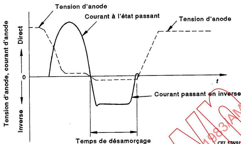
Figure 70 – Temps de désamorçage après commutation du circuit
