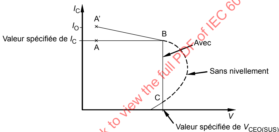
Figure 16 – Caractéristique I_C en fonction de V_{CE}
