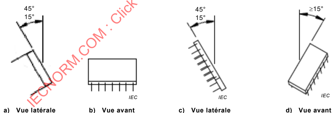
Figure 1 – Boîtiers DIP avec les conducteurs fixés aux côtés du boîtier, ou bien qui en sortent (tels que des boîtiers à brasage latéral et des boîtiers DIP en céramique)
