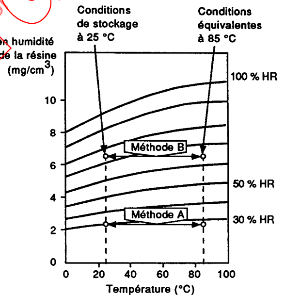
Figure 8 – Teneur en humidité saturée de la résine en fonction de la température
