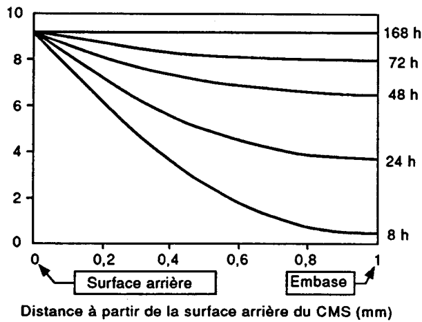
Figure 5 – Processus de diffusion de l'humidité à 85 °C, 85 % HR
