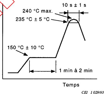
Figure 9 – Profil de température de refusion infrarouge
