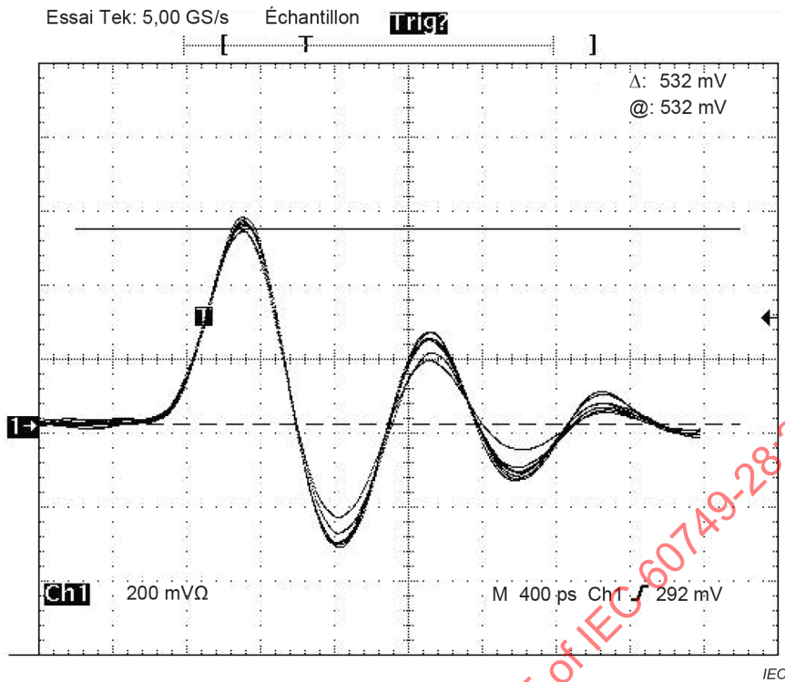
Figure F.1 – Petit module de vérification TC 500 à 1 GHz
