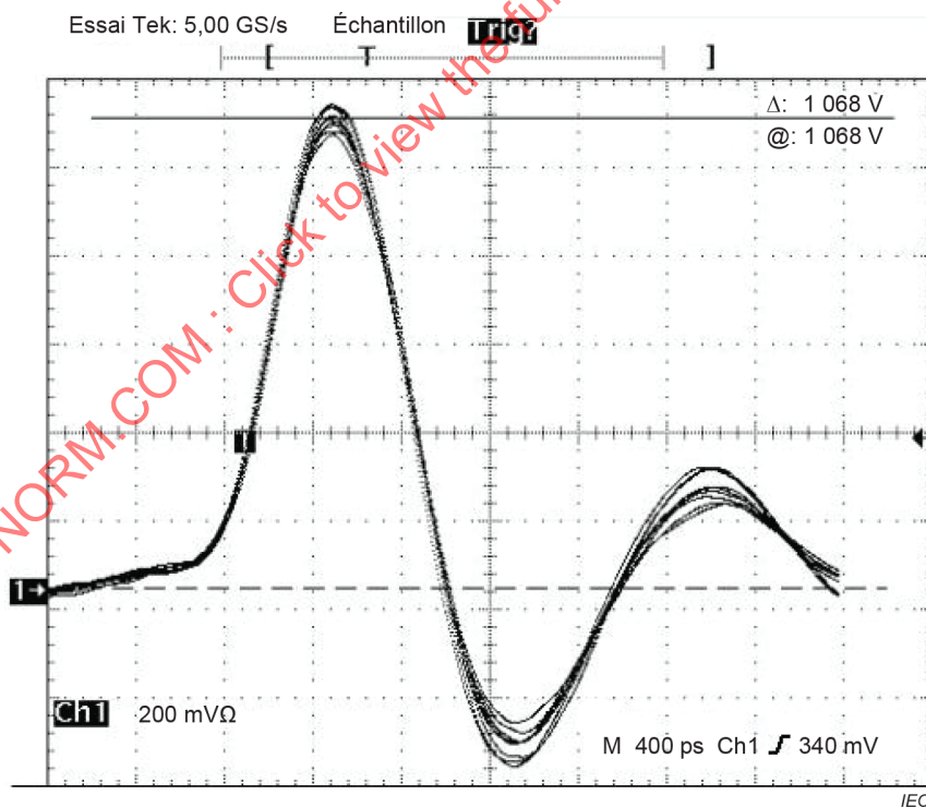
Figure F.2 – Grand module de vérification TC 500 à 1 GHz
