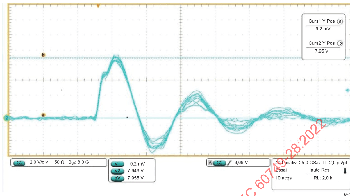
Figure F.3 – Petit module de vérification TC 500 à 8 GHz (ajustement de l'affaiblissement par l'oscilloscope)
