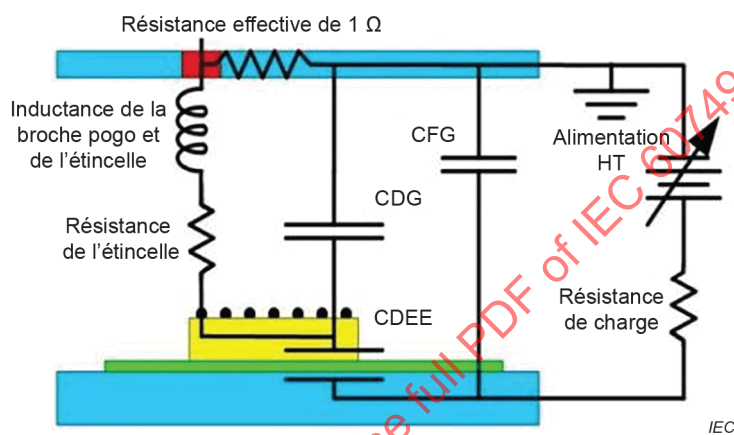
Figure E.1 – Schéma électrique simplifié de l'appareil d'essai de CDM
