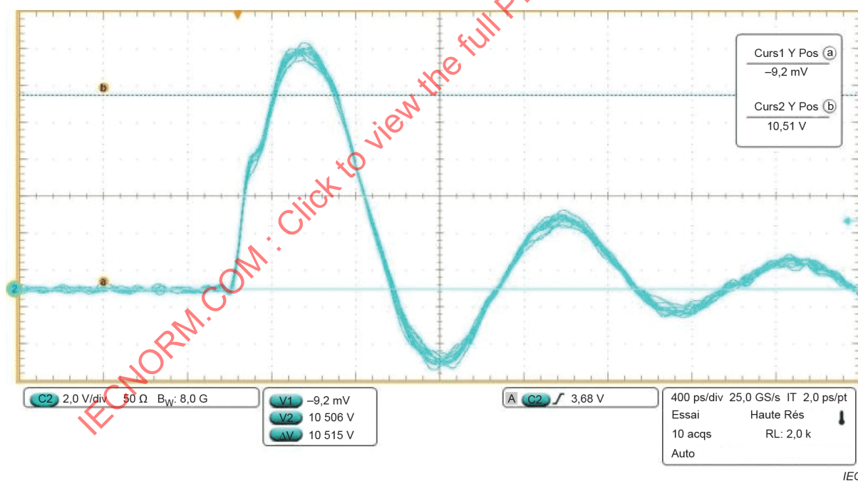
Figure F.4 – Grand module de vérification TC 500 à 8 GHz (ajustement de l'affaiblissement par l'oscilloscope)
