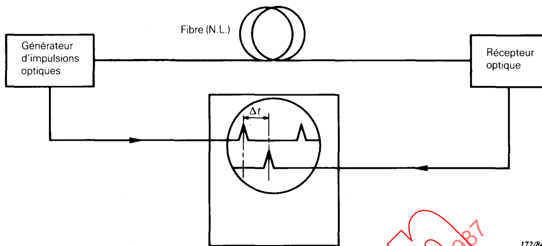
FIG. 3a. — Mesure du temps de propagation d'une impulsion transmise.
