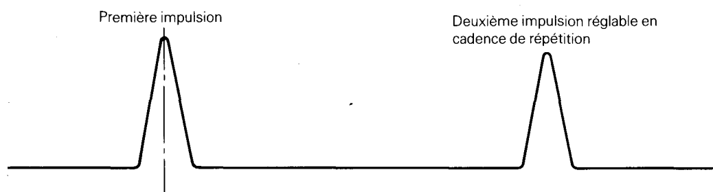
FIG. 4a. — Voie 1: impulsion émise.
