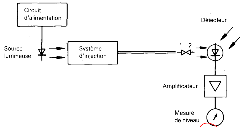
FIG. 13. — Dispositif d'étalonnage de la mesure des pertes d'insertion.
