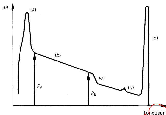
FIG. 16. — Exemple de courbe de puissance rétrodiffusée.
