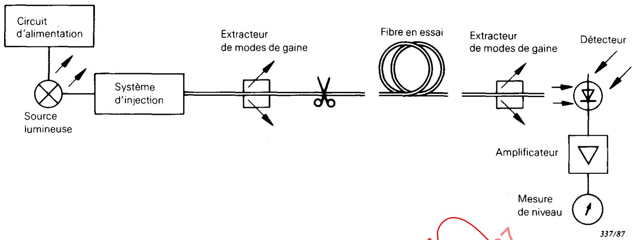
FIG. 11. — Appareillage de mesure de l'affaiblissement à une longueur d'onde spécifiée.
