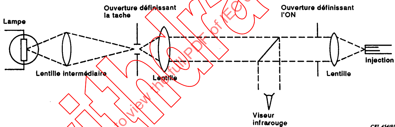
Figure 11B - Appareillage de mesure de l'affaiblissement spectral
