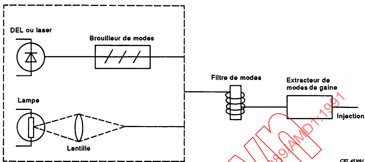
Figure 11A - Appareillage de mesure de l'affaiblissement à une longueur d'onde spécifiée
