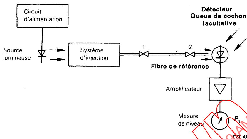
Figure 14 - Dispositif d'étalonnage de la mesure des pertes d'insertion
