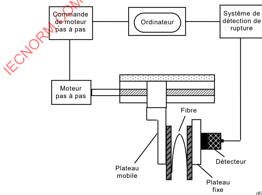
Figure B.1 – Schéma de l'appareil de courbure en deux points
