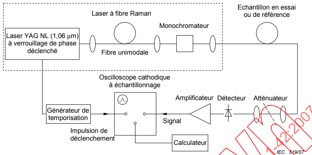
Figure B.1 – Schéma fonctionnel, système laser à fibre Raman
