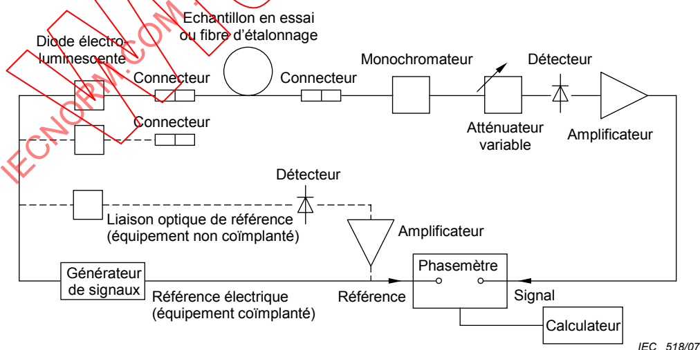
Figure A.3 – Montage de mesure de dispersion chromatique, système à diodes électroluminescentes (exemple type)
