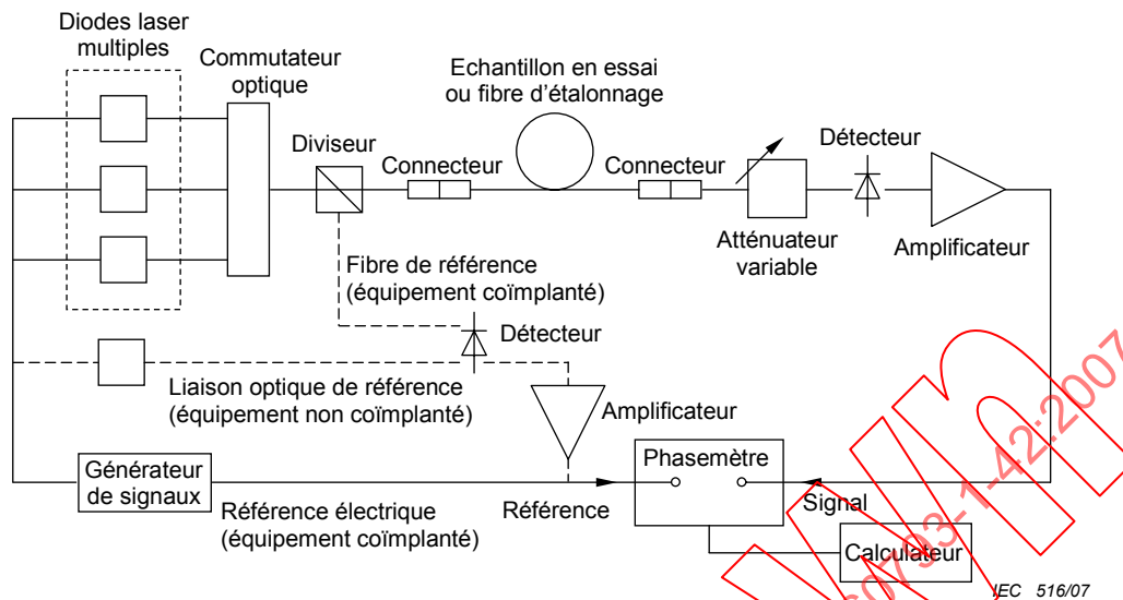
Figure A.1 – Montage de mesure de dispersion chromatique, système à diodes laser multiples (exemple type)
