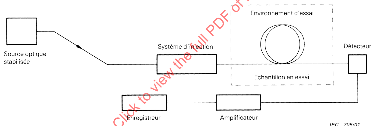
Figure A.2 – Mesure des variations du facteur de transmission optique en utilisant une source stable
