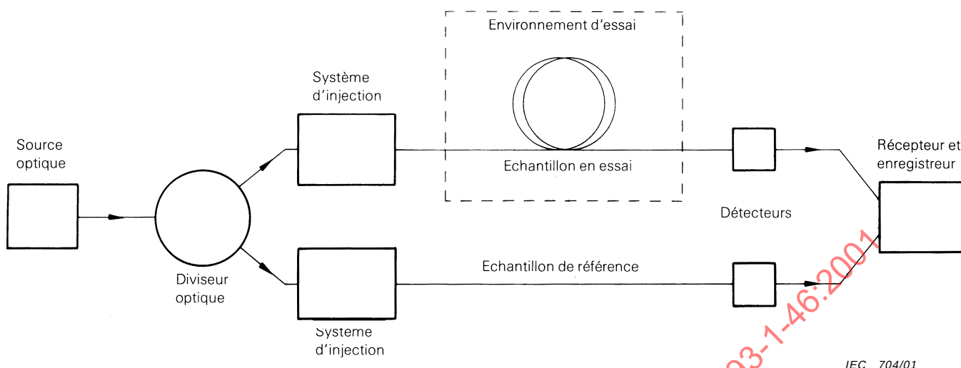
Figure A.1 – Mesure des variations du facteur de transmission optique en utilisant un échantillon de référence
