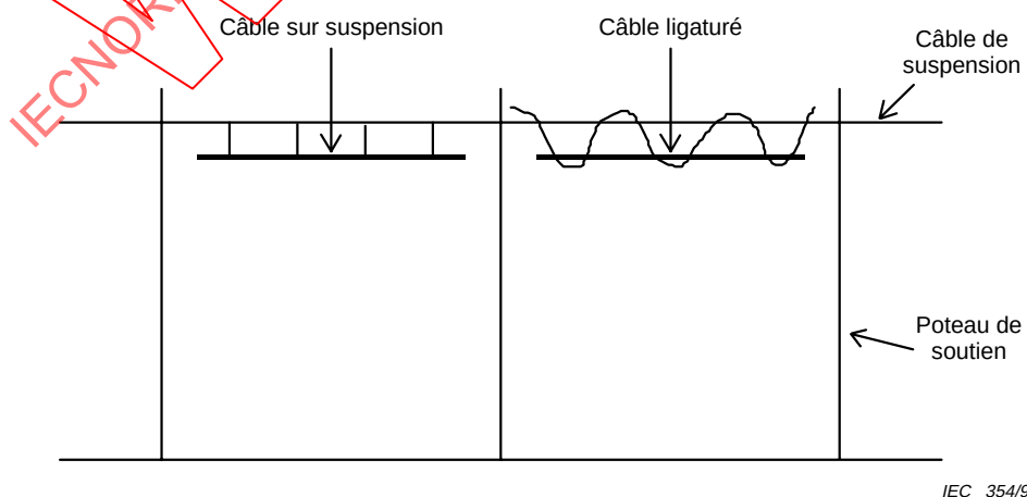
Figure C.3 – Installation de câble aérien
