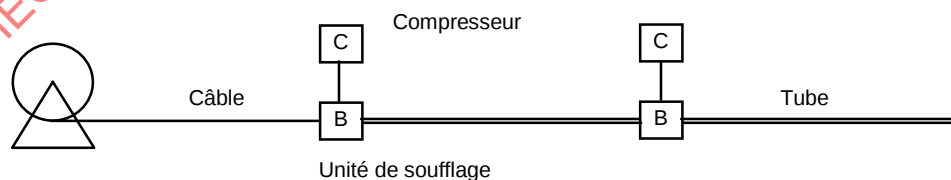
Figure A.4 – Installation de câble par soufflage en cascade
