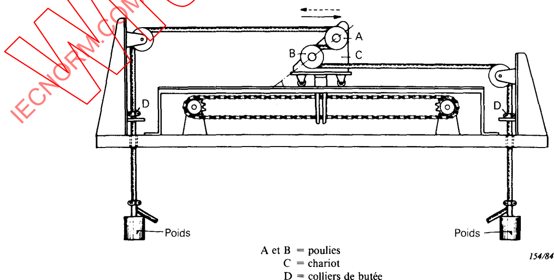
FIG. 4. — Appareil pour l'essai de flexions alternées.
