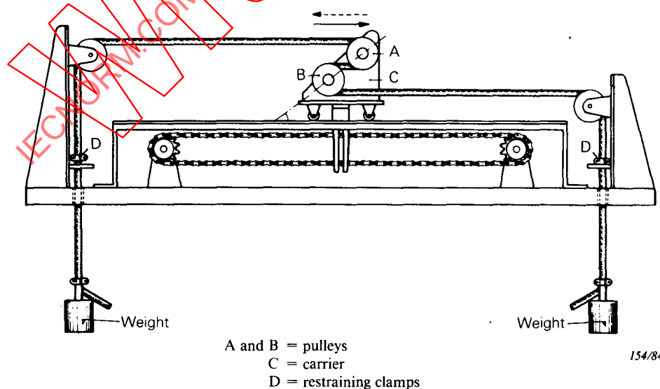
FIG. 4. — Flexing apparatus.
