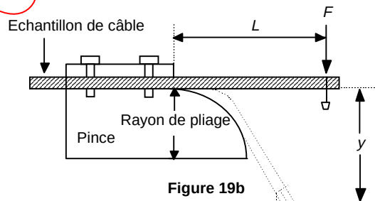
Figure 19 – Méthode E17B – Montage d'essai
