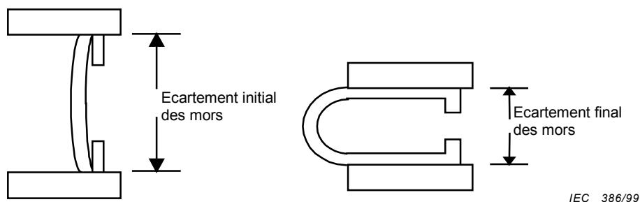
Figure 23 – Méthode E17C – Montage d'essai
