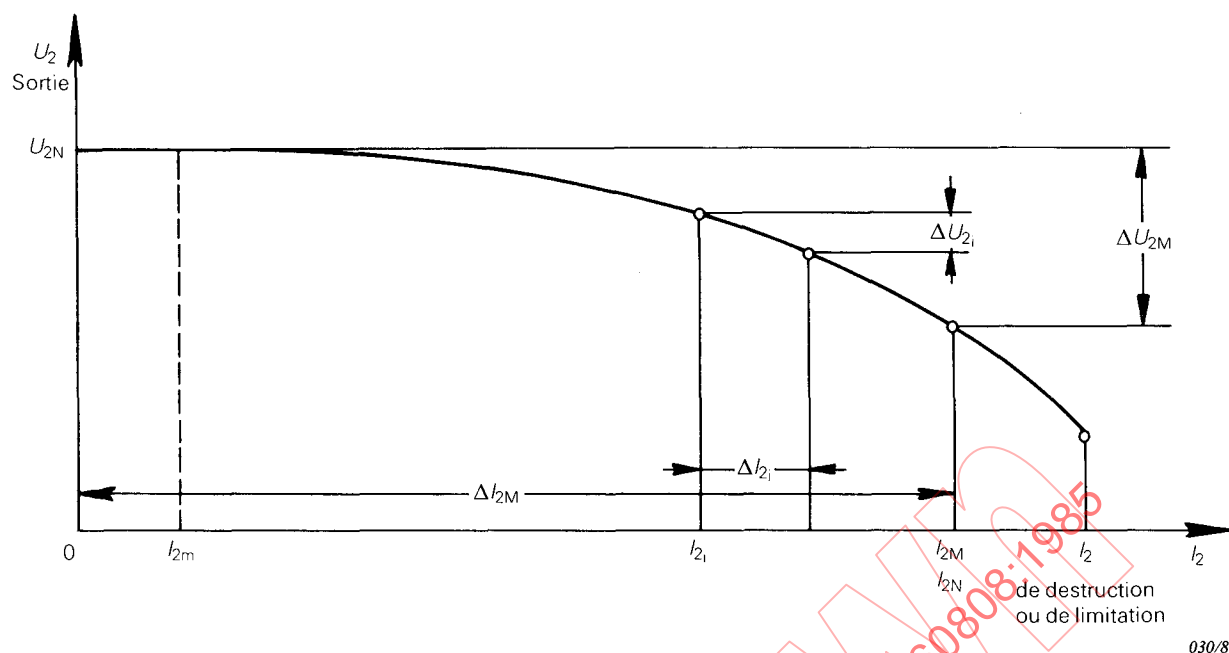
FIG. 6. — Variations en fonction de la charge.
