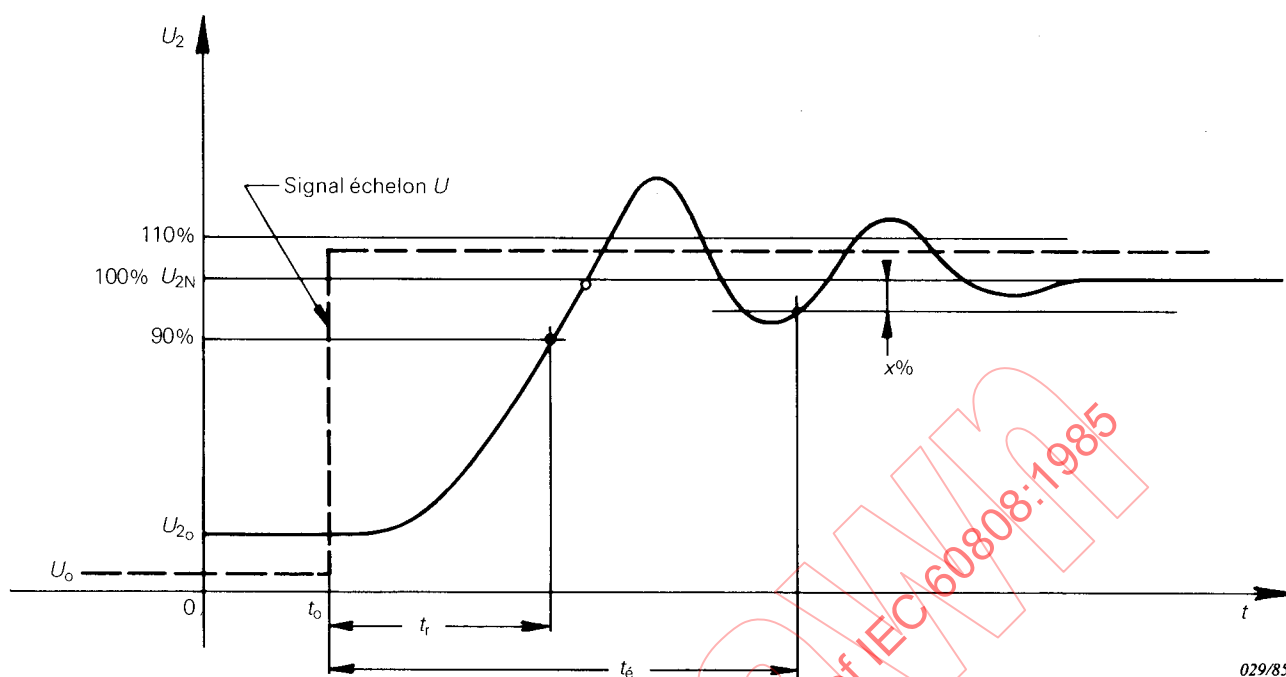
FIG. 5. — Temps de réponse.
