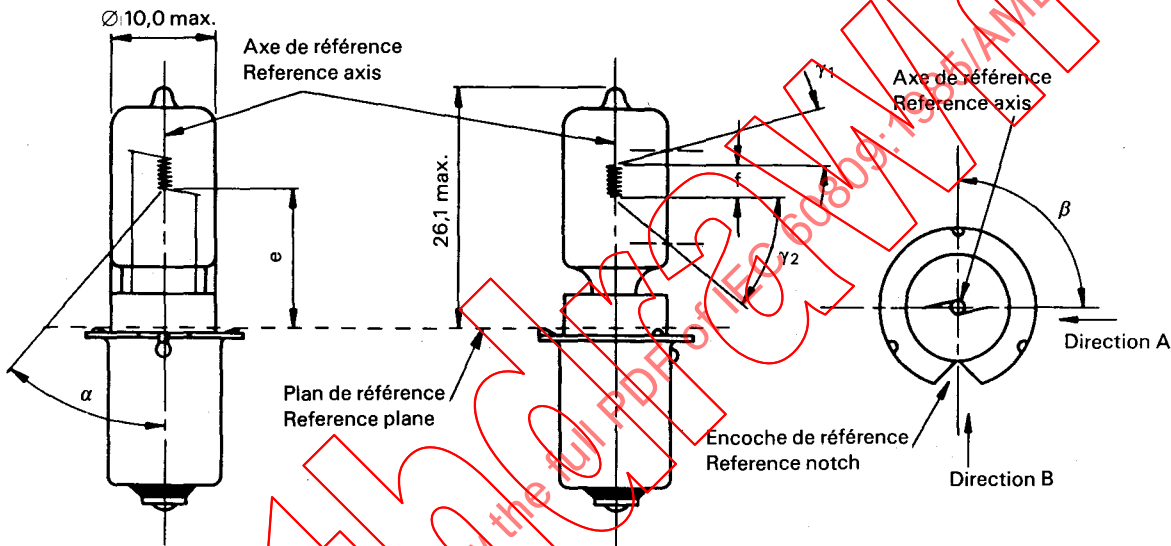
Dessin de la lampe — Lamp drawing Dimensions en millimètres — Dimensions in millimetres
