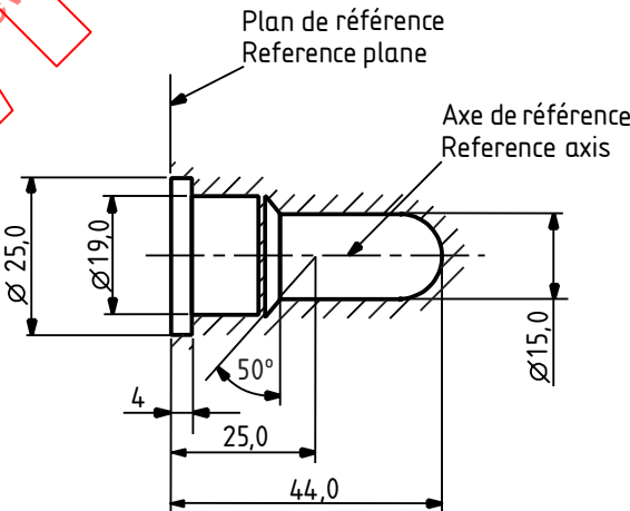
Figure 2 - Encombrement maximal de la lampe Maximum lamp outline
