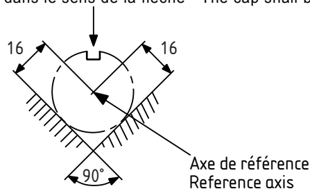
Figure 3 - Définition de l'axe de référence Definition of reference axis
