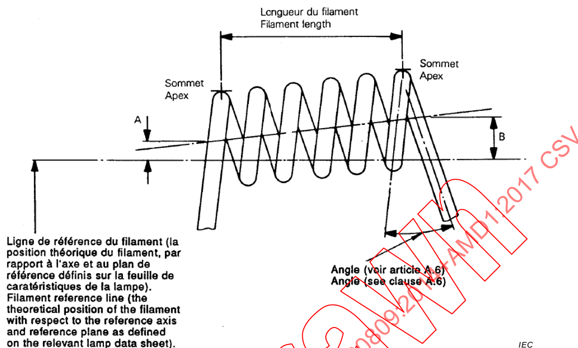
Figure A.1 – Détermination des sommets, de la longueur du filament et des décalages du filament (A et B)
