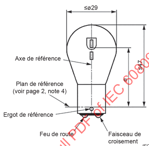
Figure 1 – Dessin de la lampe à filament
