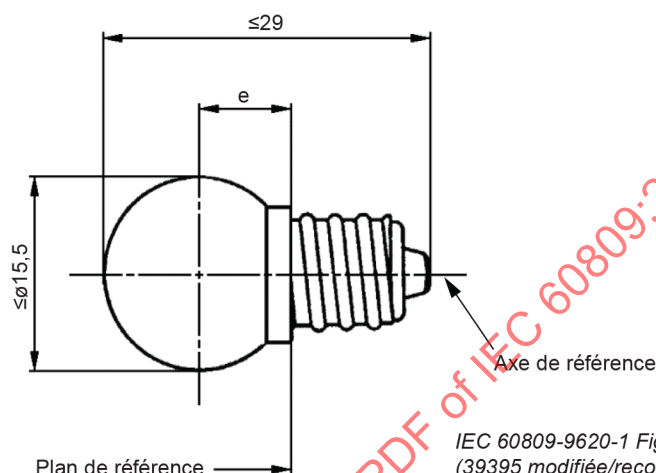
Figure 1 – Dessin de la lampe à filament Dimensions en millimètres
