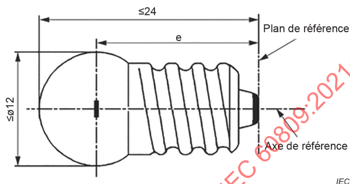
Figure 1 – Dessin de la lampe à filament Dimensions en millimètres
