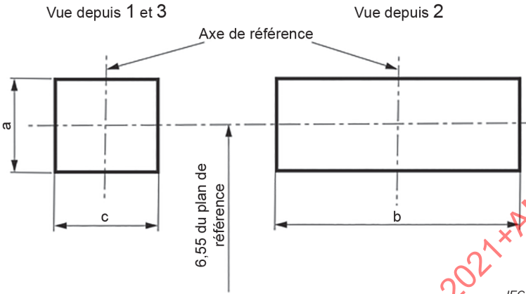
Figure 3 – Système de vérification de la localisation du filament (système de boîtier) (voir Article A.10, Annexe A) Dimensions en millimètres
