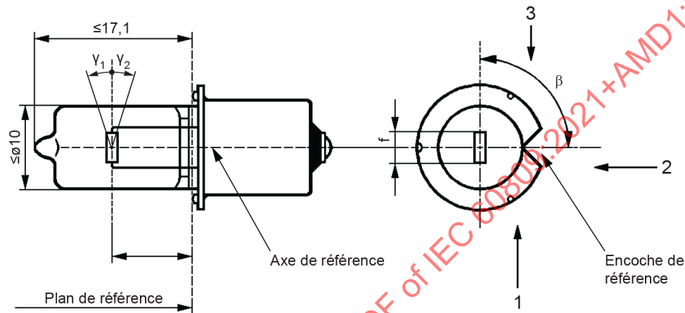
Figure 1 – Dessin de la lampe à filament
