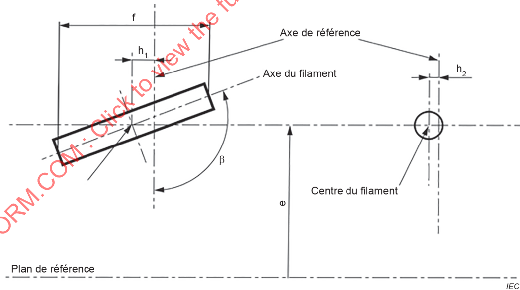
Figure 2 – Vue du filament indiquant les dimensions e, f, h_1 et h_2
