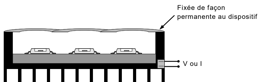
Figure 5 – Exemple de source lumineuse à LED non remplaçable
