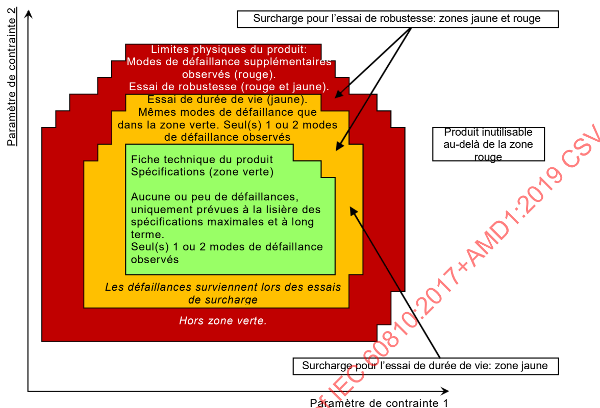
Figure M.1 – Concept de l'essai de surcharge pour deux paramètres d'essai
