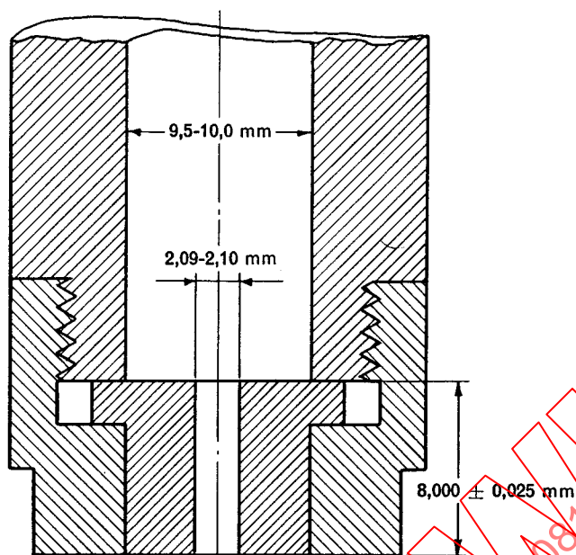
FIG. 9. — Filière (montrant le cylindre de petit diamètre extérieur et un exemple du montage de la filière).
