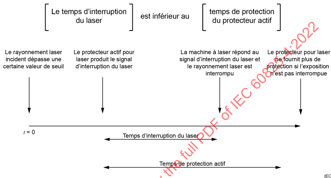
Figure C.2 – Représentation des paramètres des protecteurs actifs pour laser
