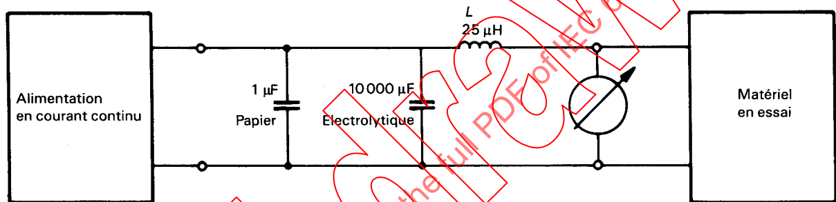
FIG. 11. — Circuit d'essai pour la mesure du bruit réinjecté.
