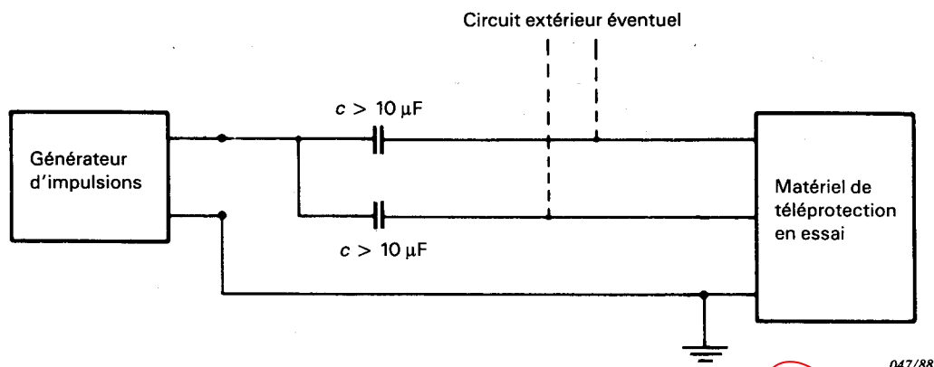
FIG. 7. — Schéma du circuit pour l'essai de tenue aux chocs en mode commun avec isolement en courant continu du générateur d'impulsions.
