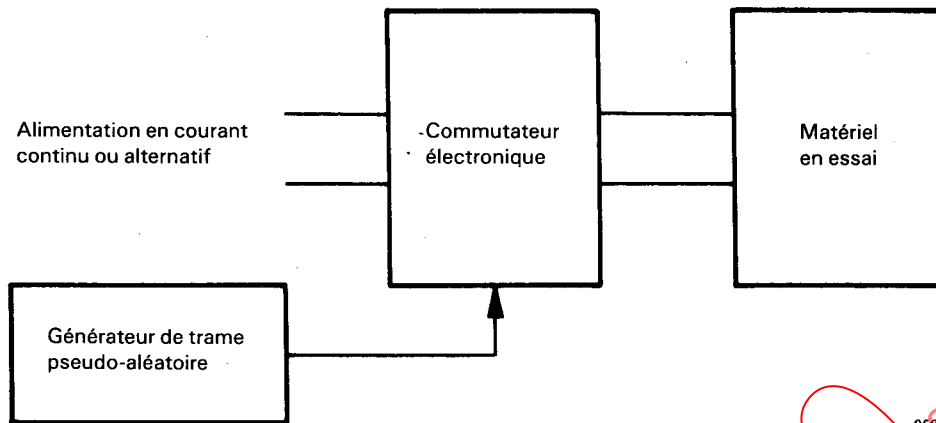
FIG. 10. — Circuit pour l'essai des interruptions d'alimentation.
