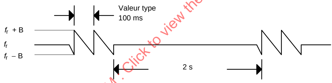
Figure 18 – Écart de fréquence en fonction du temps pour le montage de la figure 17
