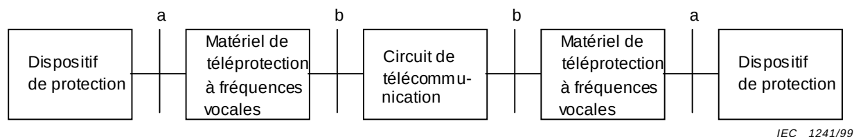
Figure 1 – Configuration de transmission à fréquences vocales
