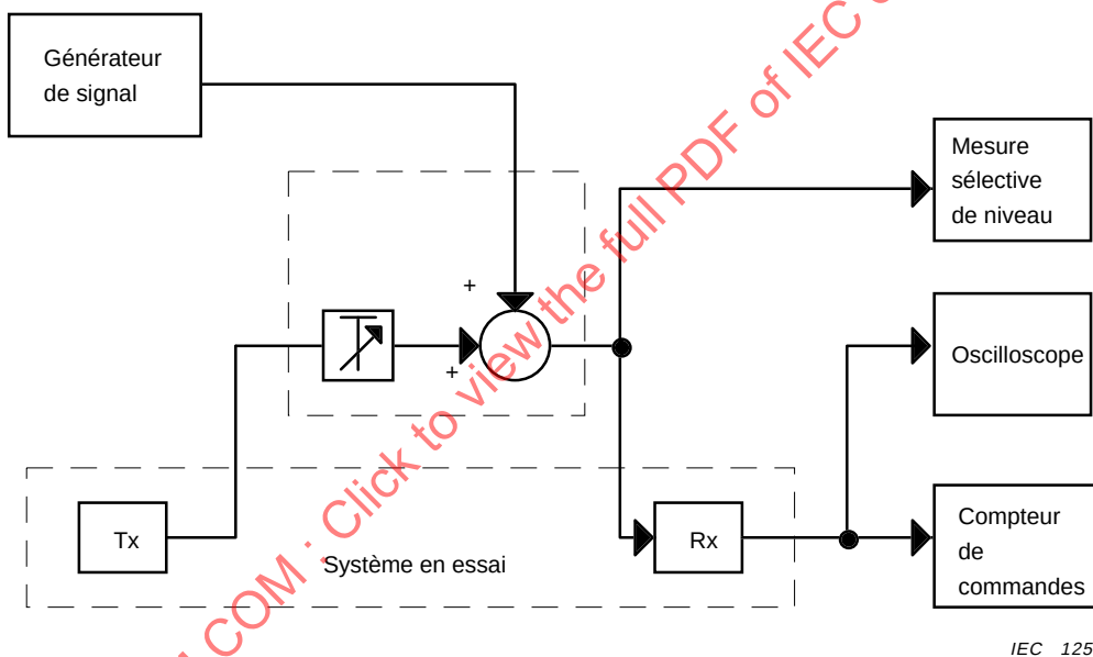
Figure 16 – Montage d'essai pour la mesure des perturbations par fréquences discrètes
