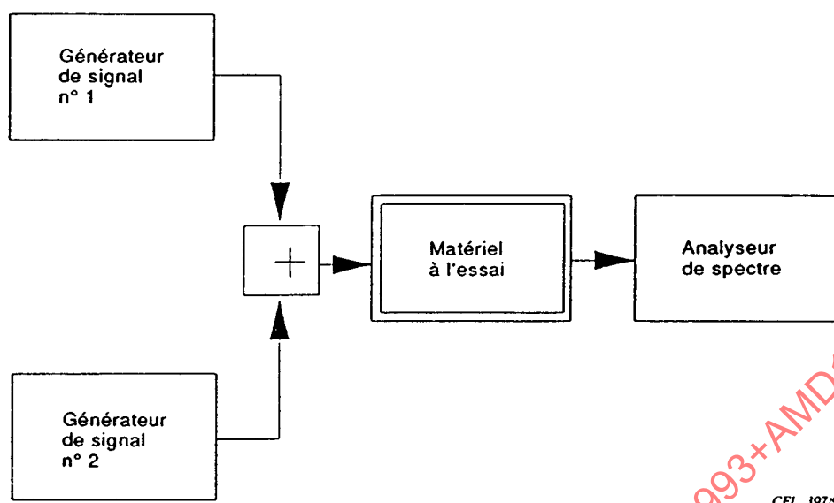
Figure 2 – Montage de mesure de la sélectivité des circuits en haute fréquence d'un récepteur de signaux numériques
