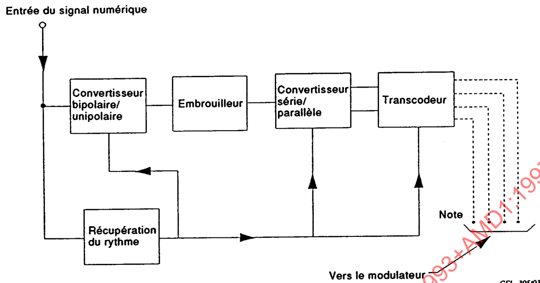
Figure 1a – Ensemble de traitement de signal d'émission
