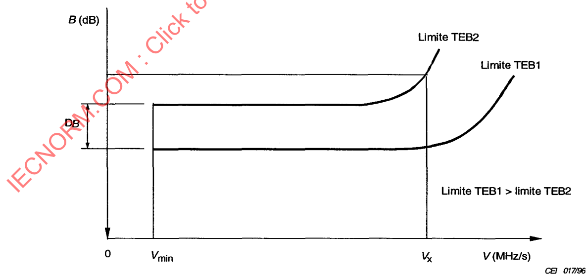
Figure 11b – Représentation graphique de la sensibilité relative du système à l'évanouissement dynamique: balayage du décalage en fréquence du creux
