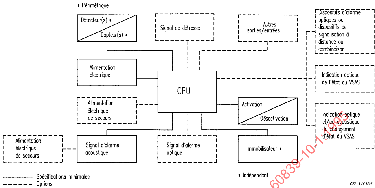
Figure 1 – Schéma bloc
