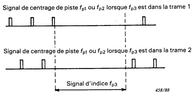
FIG. 8. — Relation entre f_{p1} , f_{p2} et f_{p3} .
