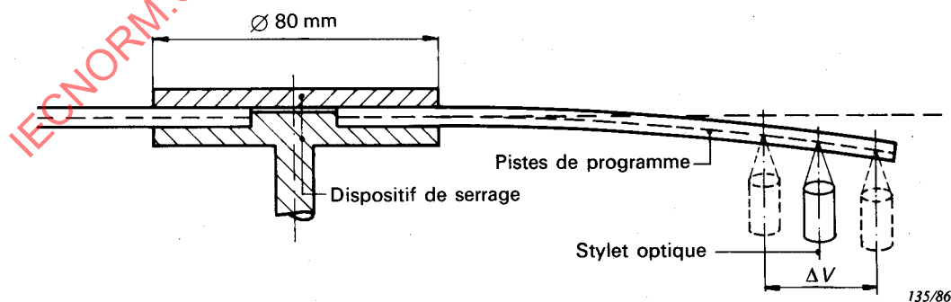
FIG. 4. — Mesure de la déviation radiale des pistes de programme au cours de la rotation à la vitesse de lecture.* Le disque est en rotation autour du centre géométrique du trou central (paragraphe 4.18).
