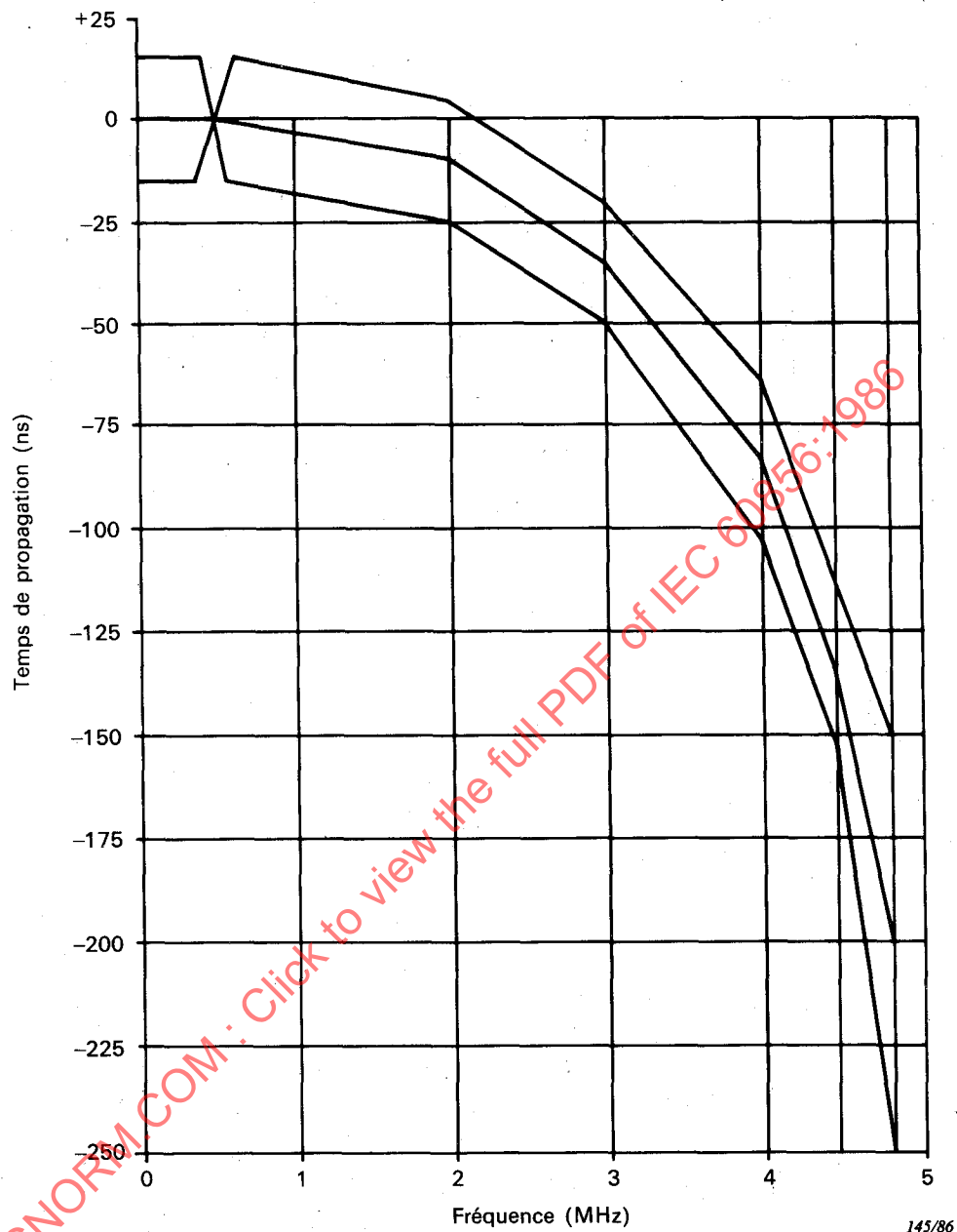
FIG. 11. — Prédistorsion du temps de propagation de groupe (paragraphe 9.1.6).
