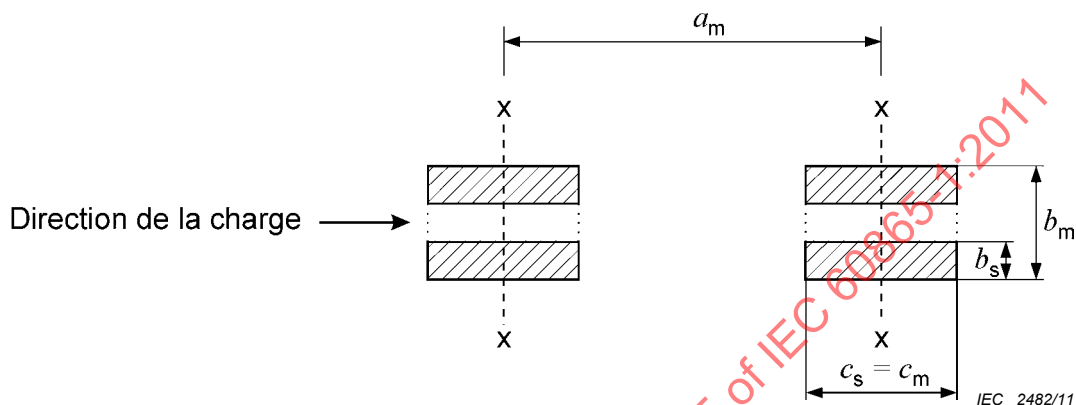
Figure 2a – Direction de la charge parallèle à la surface
