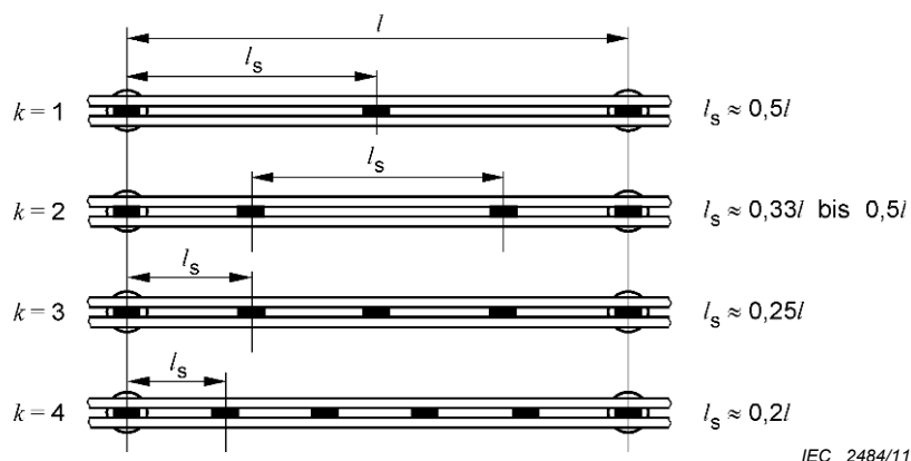
Figure 3a – Disposition des pièces de liaison dans la portée
