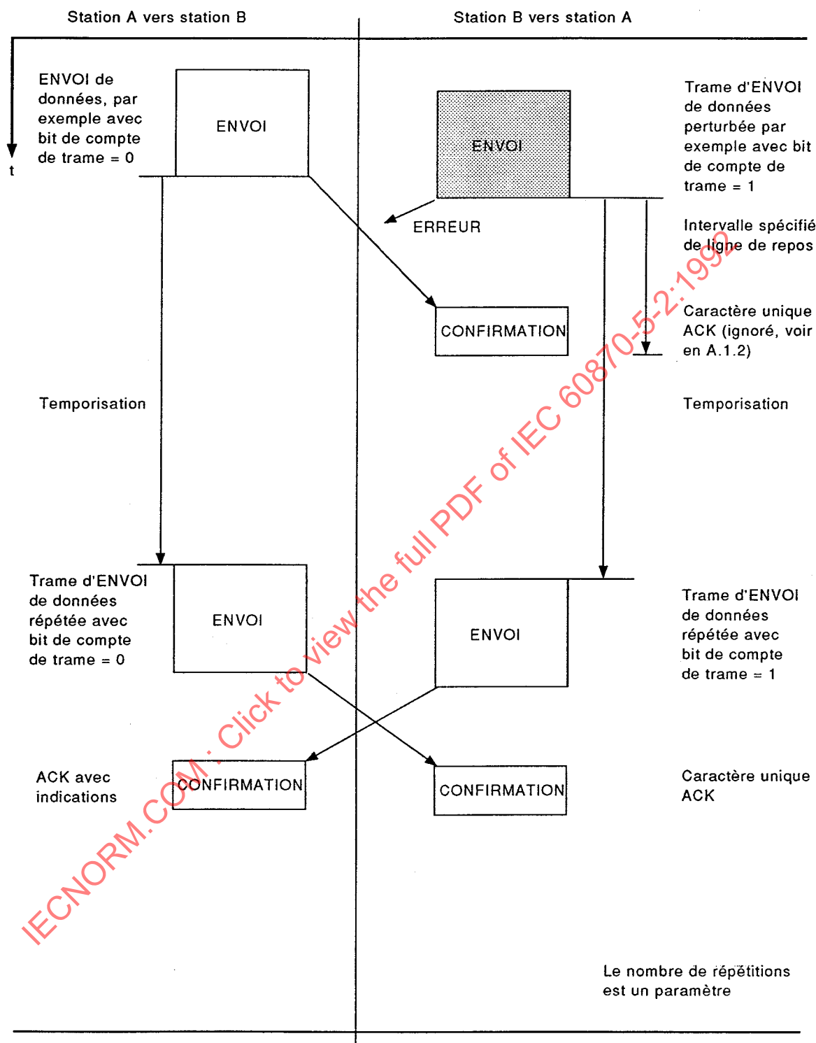
Figure 14 – Procédures de transmission équilibrées, frame ENVOI perturbée et frame de CONFIRMATION ignorée
