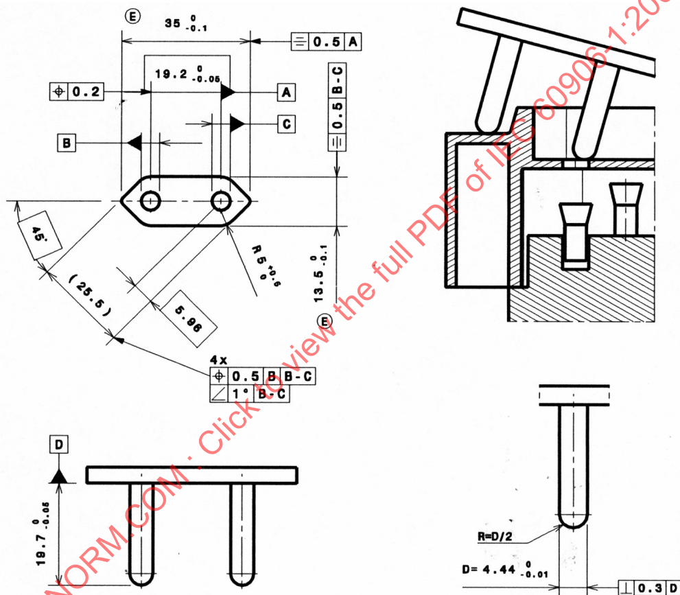
SYSTÈME DE PRISES DE COURANT 16A 250V C.A. CALIBRE POUR VÉRIFIER L'IMPOSSIBILITÉ DE L'INTRODUCTION D'UNE SEULE BROCHE DES FICHES POINT 1 ET 2 DES FEUILLES DE NORMES 1-1, 3-1 et 3-2 (Paragraphe 10.3 de la CEI 60884-1) SYSTEM OF PLUGS AND SOCKET- OUTLETS 16A 250V A.C. GAUGE FOR CHECKING IMPOSSIBILITY OF SINGLE-POLE INSERTION ITEM 1 AND 2 OF STANDARD SHEETS 1-1, 3-1 and 3-2 (Subclause 10.3 of IEC 60884-1)
