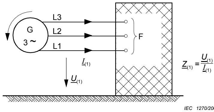
Figure 5a – Impédance de court-circuit directe \underline{Z}_{(1)}
