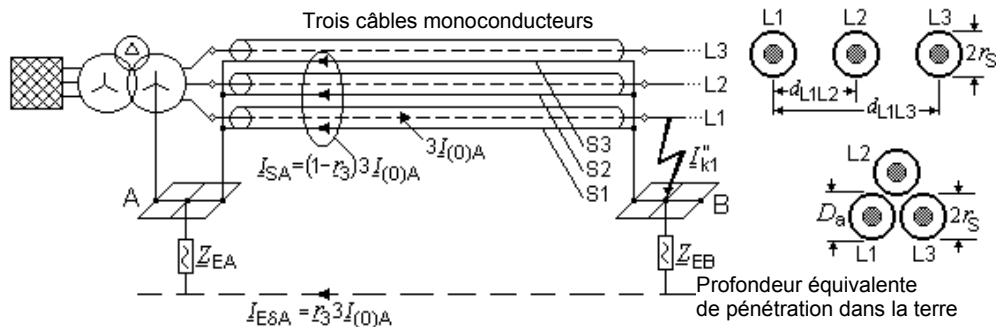
a) Alimentation à partir du poste A uniquement et court-circuit monphasé à la terre au poste B
