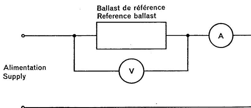
Figure 3 – Circuit d'essai type pour la mesure du rapport tension/courant du ballast de référence Recommended circuit for the measurement of voltage/current ratio of the reference ballast
