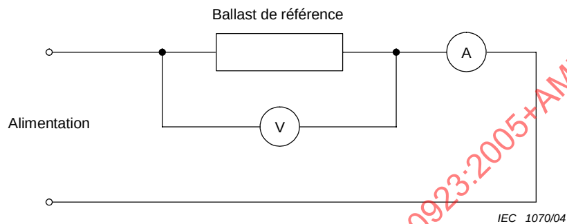
Figure A.1 – Circuit d'essai recommandé pour la mesure du rapport tension/courant du ballast de référence
