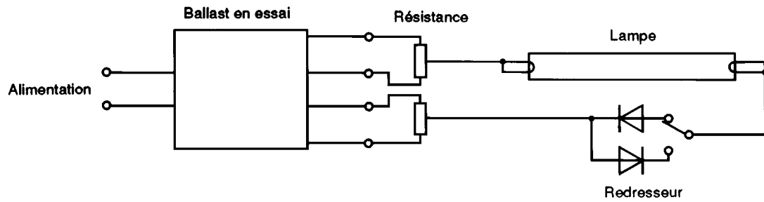
Figure 1 – Circuit pour l'essai de l'effet redresseur
