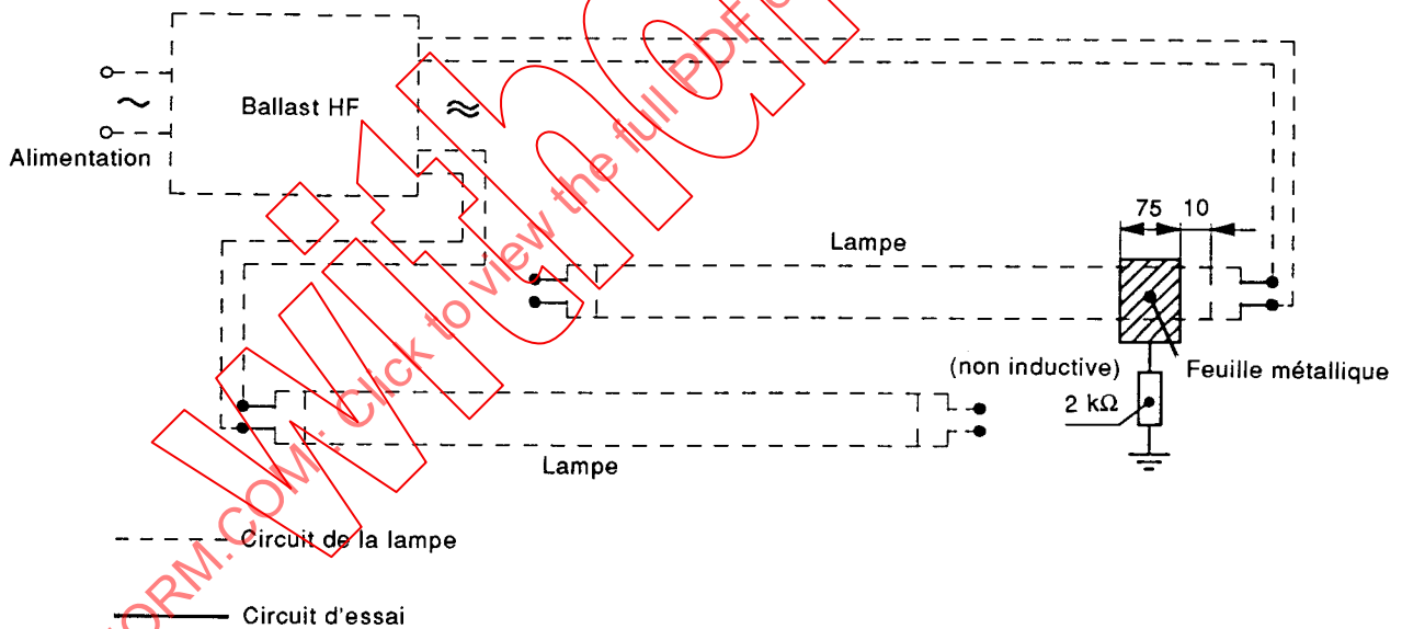
Figure 4 – Dispositif d'essai
