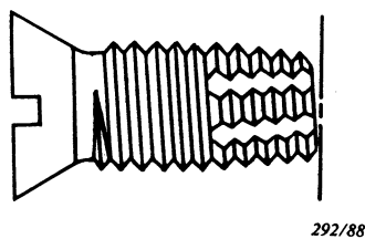
Figure 2 – Vis autotaraudeuse avec découpe
