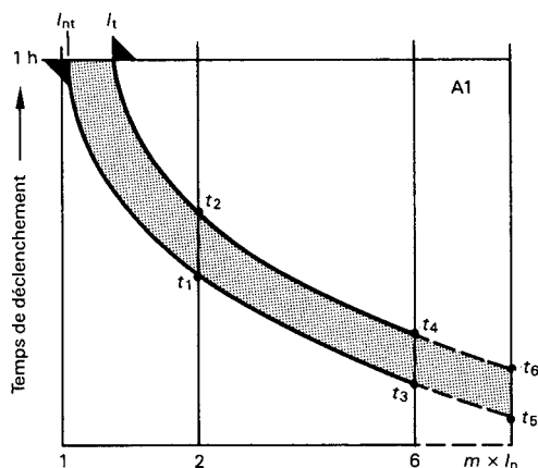
Figure A.1 – Mode thermique seul
