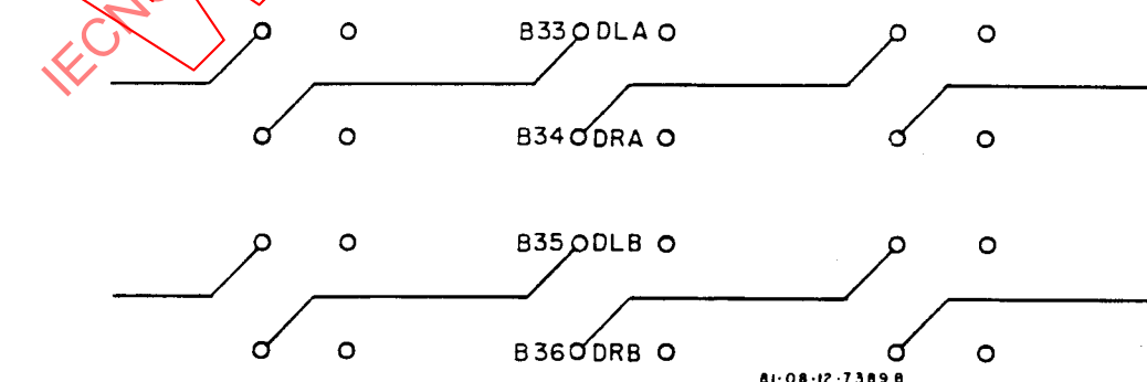
Figure 33 - CÂBLAGE DE LA GUIRLANDE DU FOND DE PANIER (VU DU DEVANT DU CHÂSSIS)
