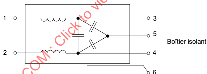
Essai A entre 1 et 2 ou 3 et 4 Essai B entre 1, 2, 3, 4 ensemble et 5 Essai C 1, 2, 3, 4, 5 ensemble et la feuille de métal 6 enroulée autour du boîtier
