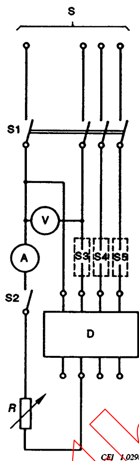
Figure B.3 – Circuit d'essai pour vérification du comportement des DPR classifiés selon B.3.1.2.2.1 (voir B.8.9)
