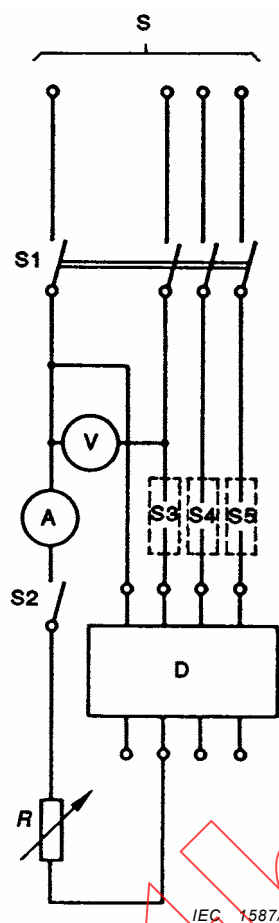
Figure B.3 – Circuit d'essai pour la vérification du comportement des DPR classifiés selon B.3.1.2.2 (voir B.8.9)
