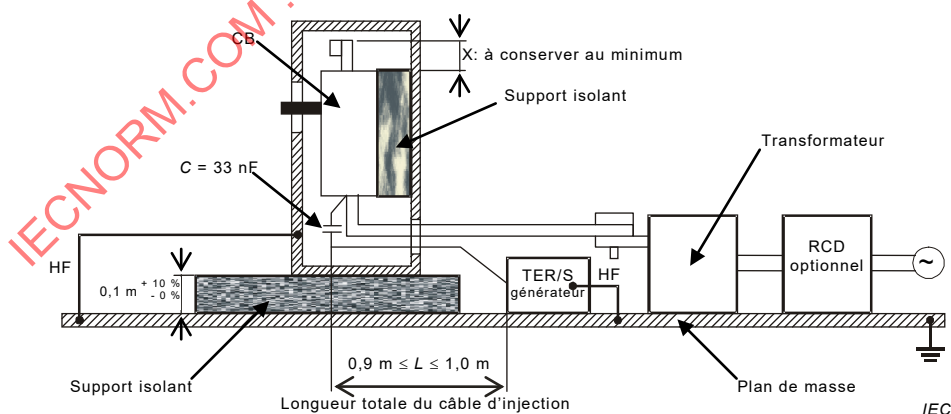
Figure F.17 – Installation d'essai pour la vérification de l'immunité aux champs électromagnétiques rayonnés aux fréquences radioélectriques
