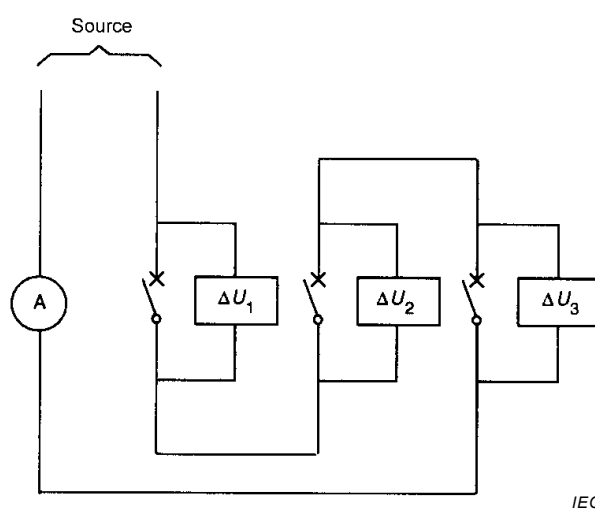
Figure G.2 – Exemple de mesurage de la perte de puissance selon G.2.2 et G.2.3
