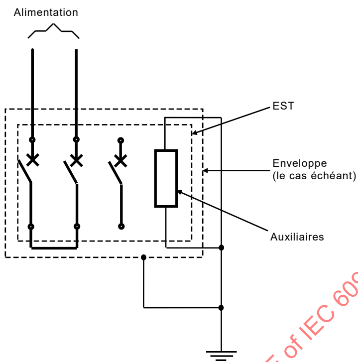
Figure F.2 – Circuit d'essai pour les essais d'immunité et d'émission selon F.4.1.3, F.4.2, F.4.3, F.4.6, F.4.7.1, F.5.4 et F.6.3 – Deux pôles de phase en série
