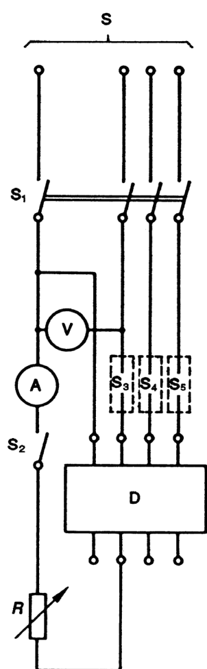
Figure B.3 – Circuit d'essai pour la vérification du comportement des DPR classés selon B.3.1.2.2 (voir B.8.9)
