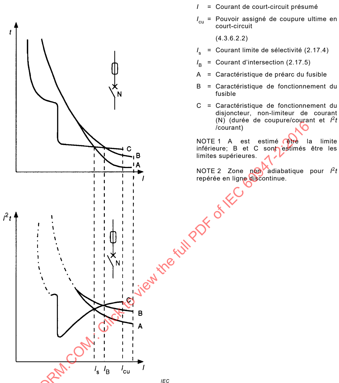
Figure A.1 – Coordination pour la surintensité entre un disjoncteur et un fusible ou protection d'accompagnement par un fusible: caractéristiques de fonctionnement
