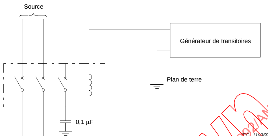
Figure 6 – Circuit d'essai pour la vérification de l'influence des transitoires dans les circuits auxiliaires (mode commun)
