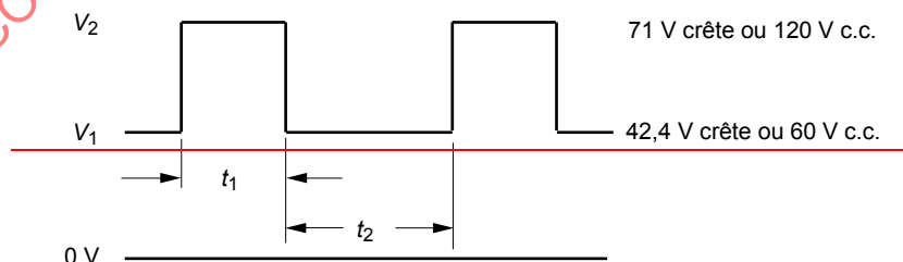
Figure 2E — Tensions dans les circuits TBTS dans les conditions de premier défaut
