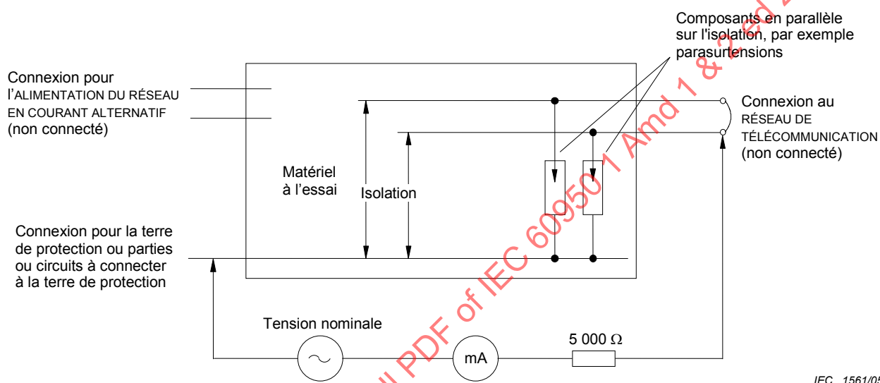
Figure 6A – Essai de la séparation entre le réseau de télécommunications et la terre
